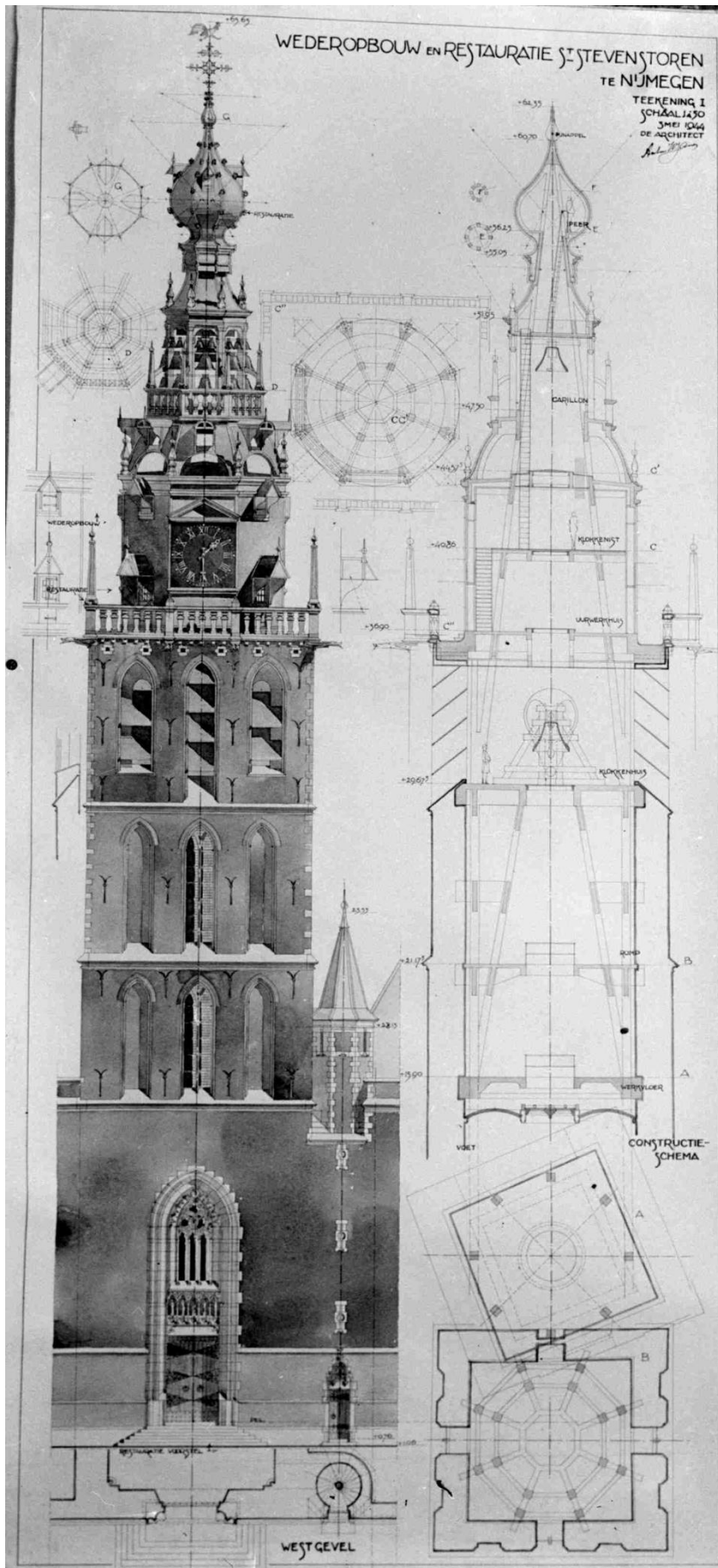
Tekening van de restauratie van de St. Stevenstoren van architect A.W. Jansz d.d. 3 mei 1944
